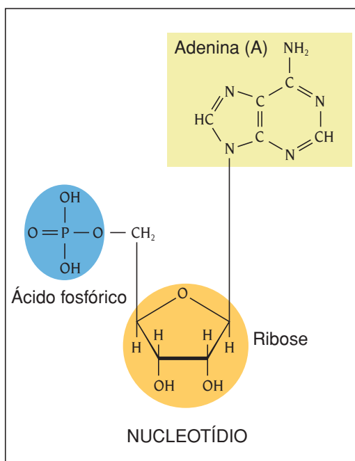
▲ Figura 3.32 • Componentes dos ácidos nucleicos. O açúcar desoxirribose e a base nitrogenada timina ocorrem exclusivamente no DNA. O açúcar ribose e a base uracila, por sua vez, são exclusivos do RNA. Os demais componentes são comuns ao DNA e ao RNA.
